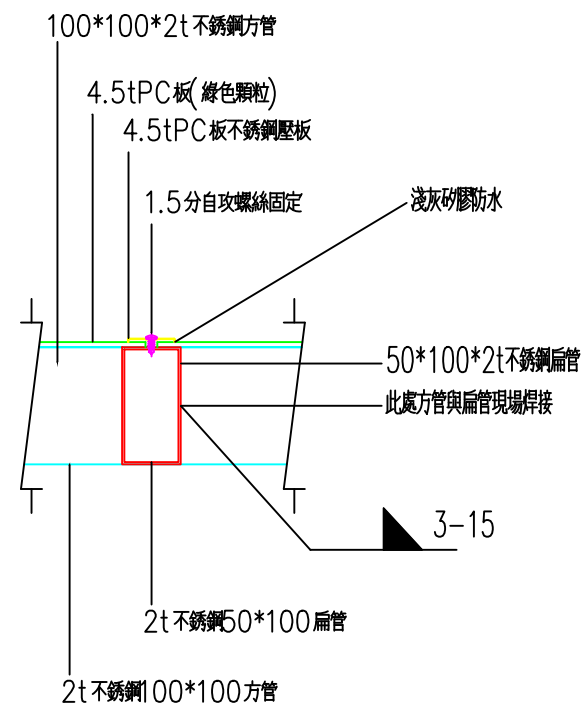
連接詳圖A
